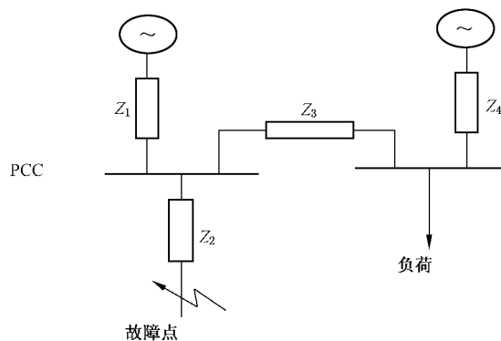
图 B.2 有负荷端自电源的供电系统的等值电路
